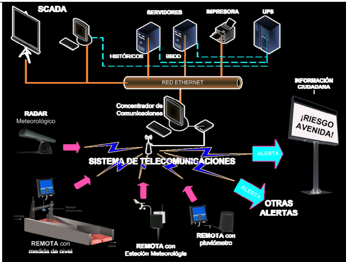
Esquema de red del sistema de alerta temprana
